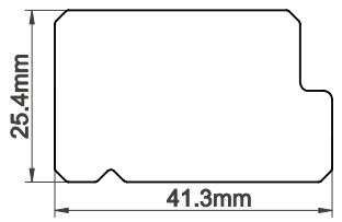
41.3mm Chamfer Rebate Stile
