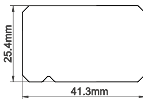
41.3mm Chamfer Butt Stile
