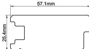
57mm Chamfer Rebate Stile
