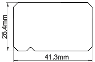
41.3mm Plain Butt Stile
