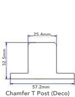
Chamfer T Post (Deco)
